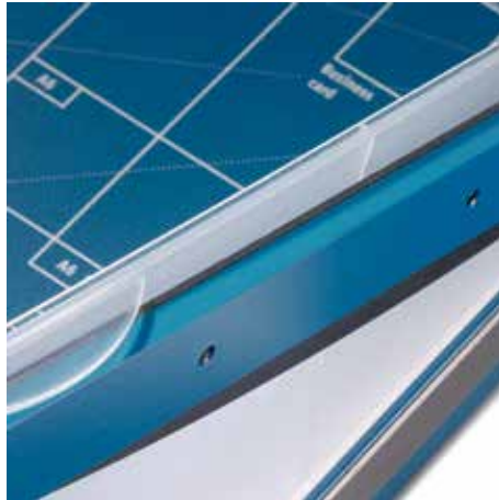
Dos de lame fixe en acier plein pour un guidage optimal de la lame supérieure vissée
